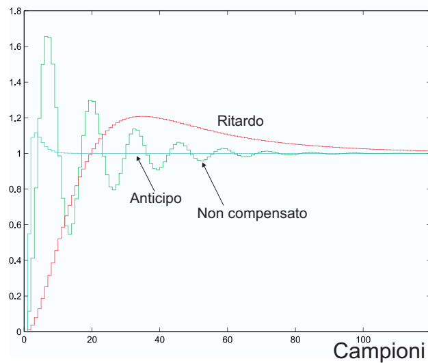
Figura 6.11: Risposta del sistema al gradino con rete anticipatrice, rete ritardatrice e senza compensazione.
