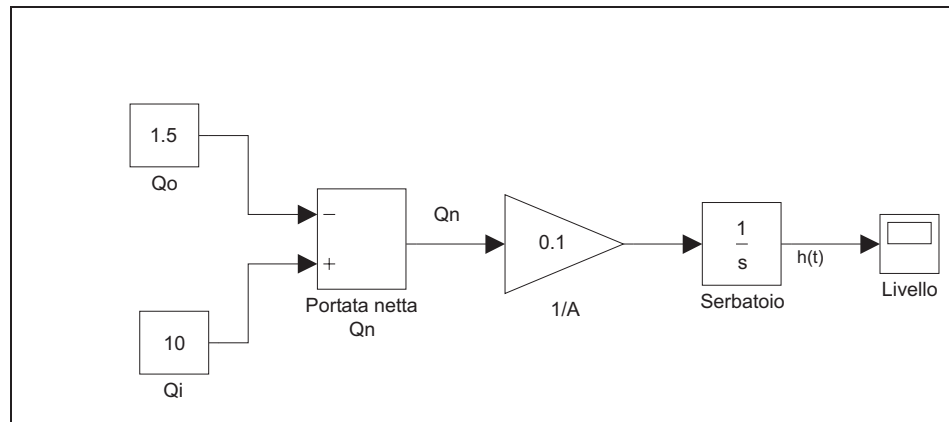
Figura 5.7: Schema Simulink del sistema controllato.
