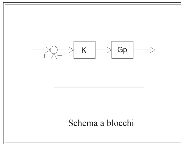
Figura 4.12: Schema a blocchi relativo al luogo delle radici per G_p(s) .
