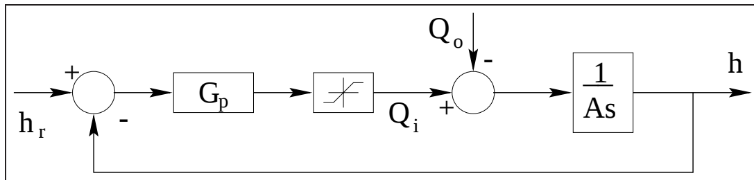
Figura 5.9: Schema a blocchi del controllo di livello con PID.
