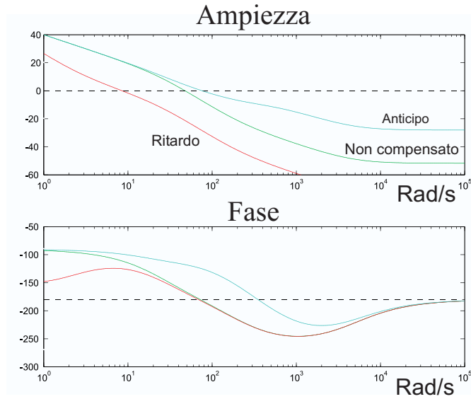
Figura 6.10: Diagrammi di Bode del sistema con rete anticipatrice, rete ritardatrice e senza compensazione.
