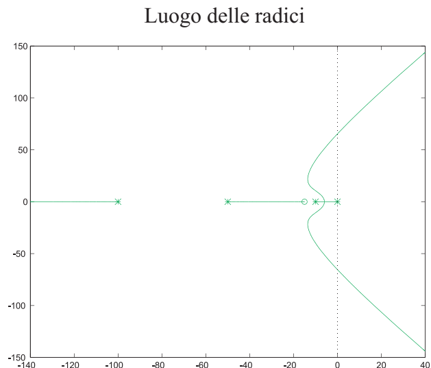
Figura 4.13: Luogo delle radici per G_c(s)G_p(s) .
