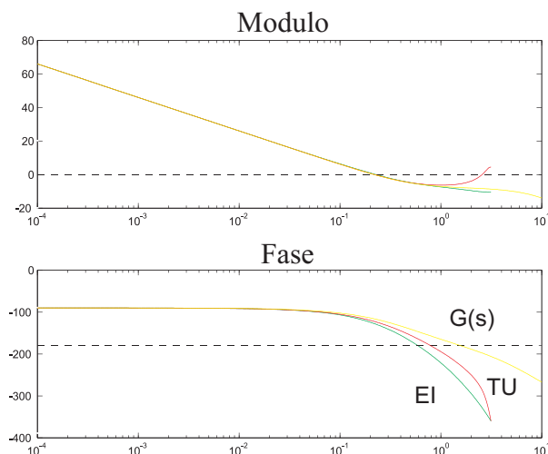
Figura 6.4: Diagrammi di bode delle funzioni d'anello.
