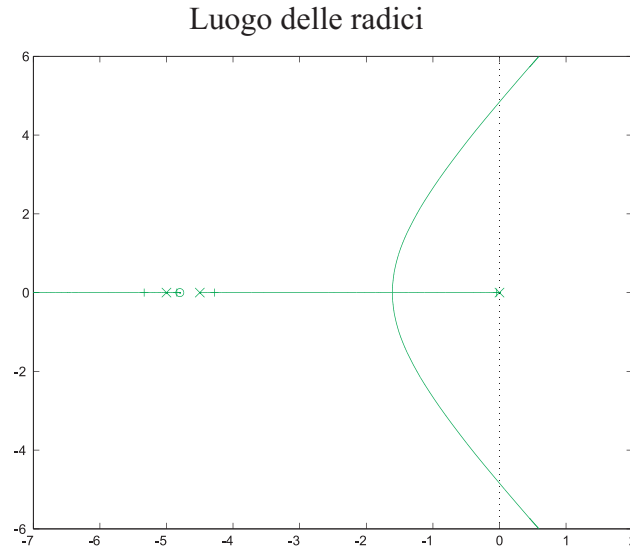
Figura 4.17: Luogo delle radici per G_{c1}G_p(s) .
