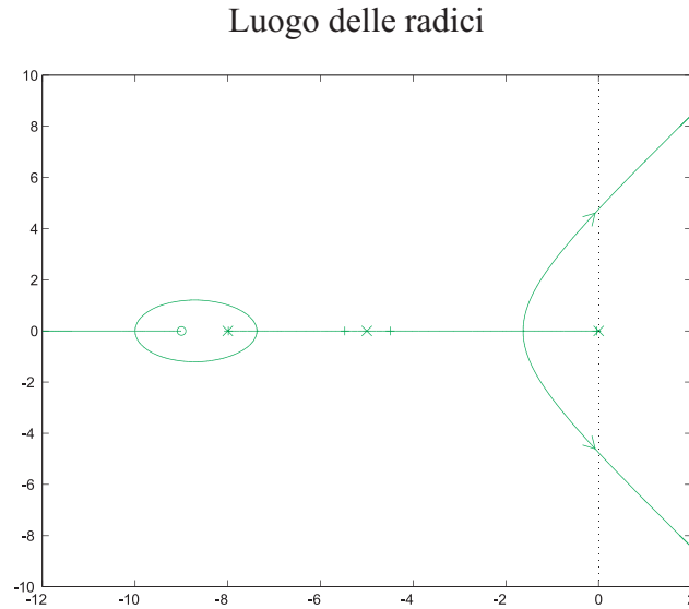
Figura 4.19: Luogo delle radici della funzione G_{c2}(s)G_p(s) .
