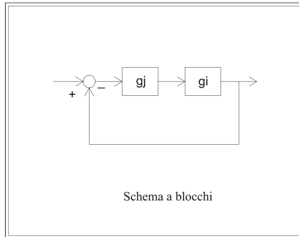
Figura 4.2: Schema in retroazione con una rete ritardatrice.
