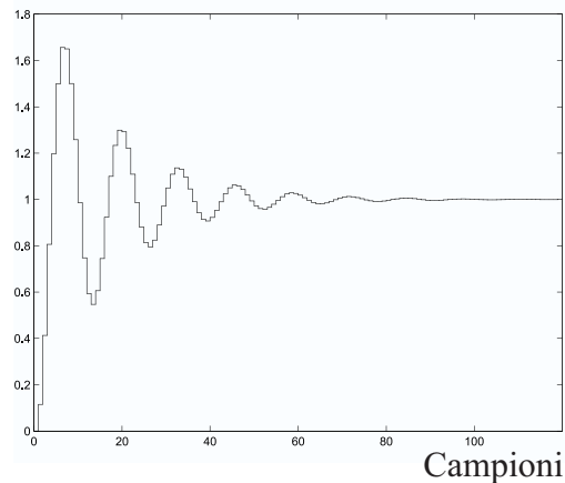
Figura 6.6: Risposta al gradino del sistema non compensato.
