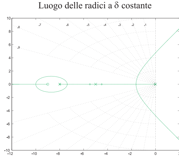
Figura 4.20: Luogo delle radici a \delta costante per la funzione G_{c2}(s)G_p(s) .
