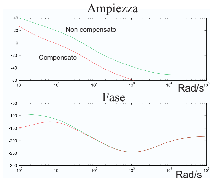
Figura 6.8: Diagrammi di Bode del sistema compensato e non compensato.
