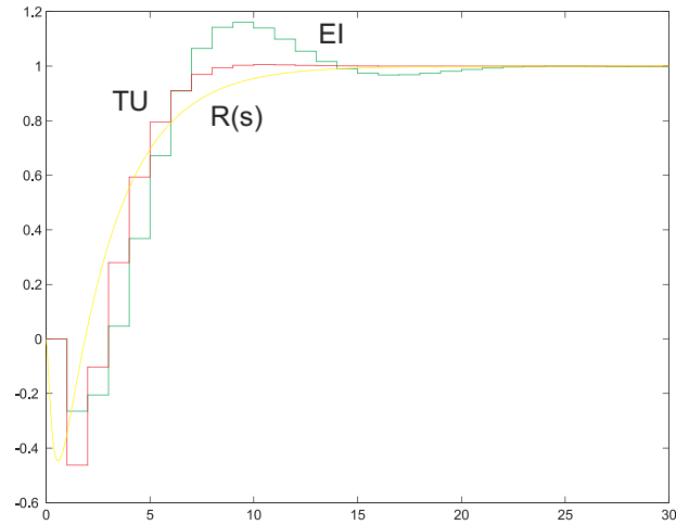
Figura 6.5: Risposta al gradino del sistema di controllo digitale.
