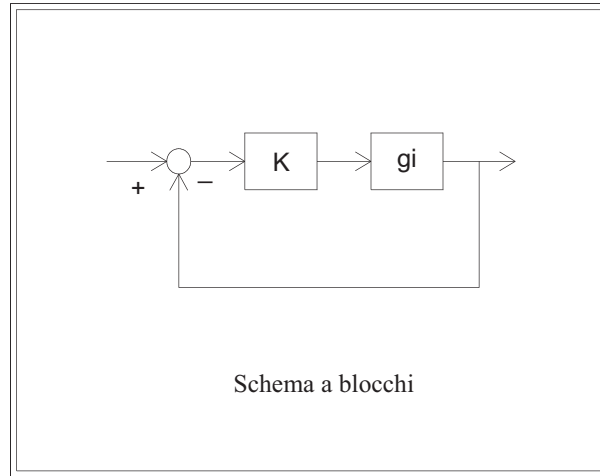
Figura 4.3: Schema per il calcolo del luogo delle radici.
