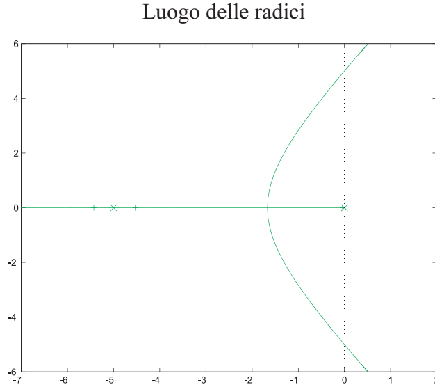
Figura 4.16: Luogo delle radici per G_p(s) .
