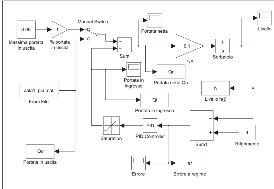
Figura 5.8: Schema Simulink del controllo di livello con PID.
