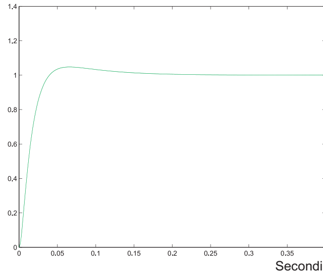
Figura 4.10: Risposta al gradino del sistema chiuso in retroazione unitaria.
