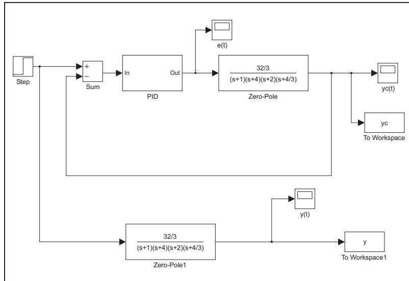
Figura 5.17: Il sistema controllato G(s) in retroazione con il PID.
