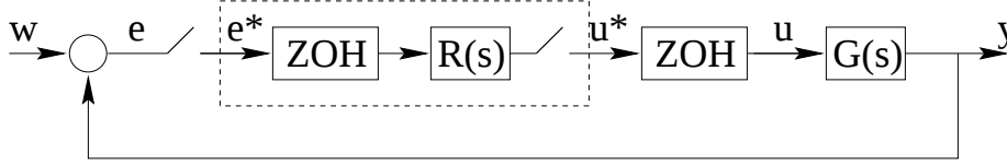
Figura 6.2: Schema equivalente del sistema di controllo digitale ottenuto con HE.
