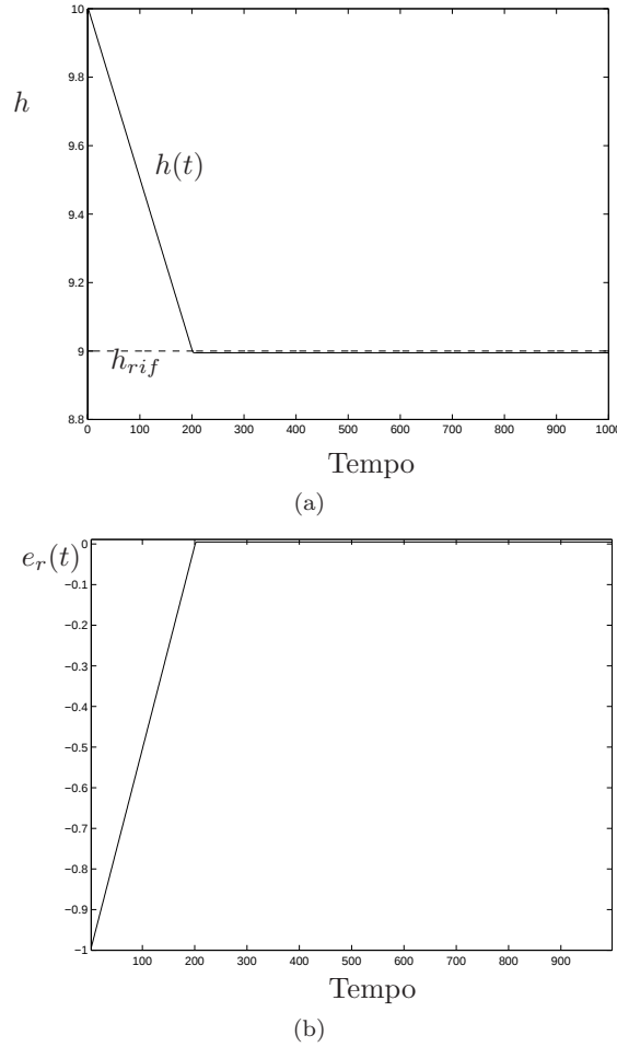
Figura 5.10: Livello del serbatoio e livello di riferimento (a) ed errore a regime (b) con regolatore P.
