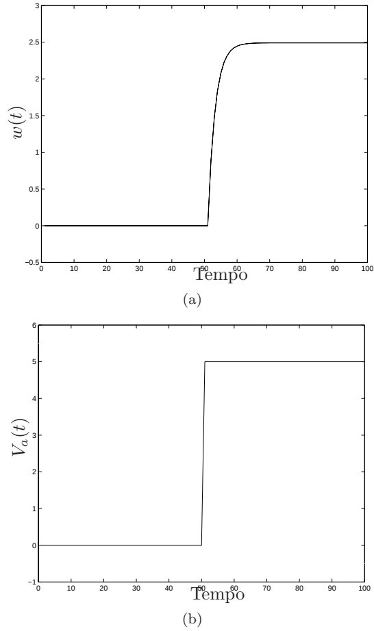
Figura 3.13: Velocità angolare del motore in cc (a) soggetto ad un gradino di tensione (b).
