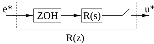
Figura 6.1: Regolatore analogico ai segnali campionati.
