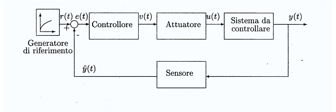
Figura 5.1: Diagrammi a blocchi di un sistema di controllo.
