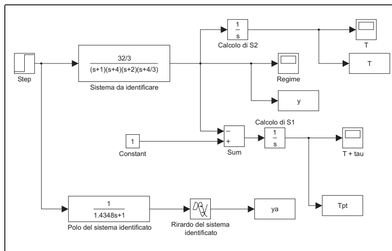
Figura 5.14: Modello Simulink per l'identificazione di G(s) .
