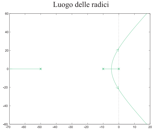
Figura 4.11: Luogo delle radici di G_p(s) .
