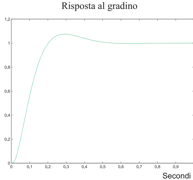
Figura 4.15: Risposta al gradino del sistema KG_c(s)G_p(s) chiuso in retroazione con K = 6000 .
