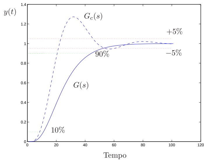
Figura 5.18: Risposte del sistema con e senza compensazione e livelli di riferimento.
