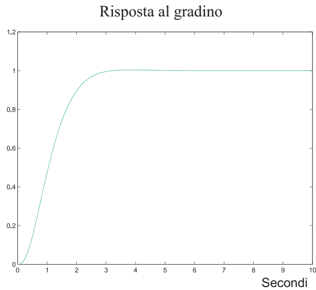
Figura 4.21: Risposta al gradino per la funzione KG_{c2}(s)G_p(s) .
