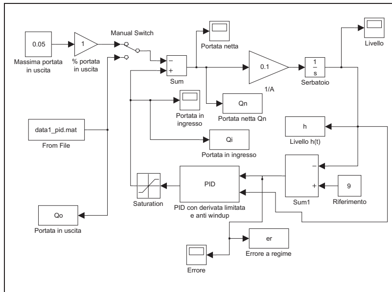
Figura 5.21: Schema Simulink di PID modificato e serbatoio.
