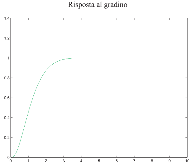
Figura 4.18: Risposta al gradino per il sistema G_1(s) = 21G_{c1}(s)G_p(s) .
