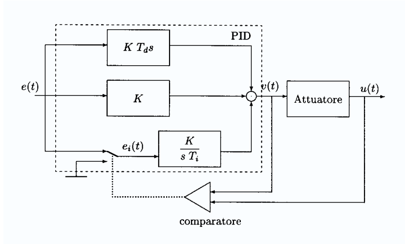
Figura 5.5: Schema di antisaturazione mediante integrazione condizionata.
