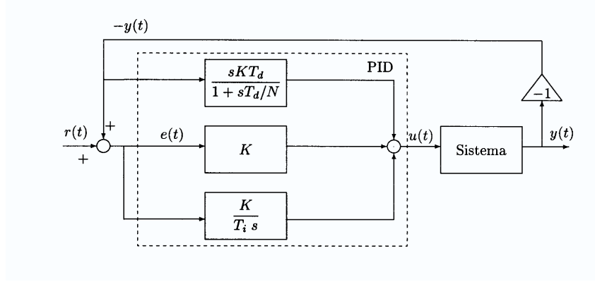
Figura 5.2: Schema a blocchi del PID con limitazione di banda del termine derivativo.
