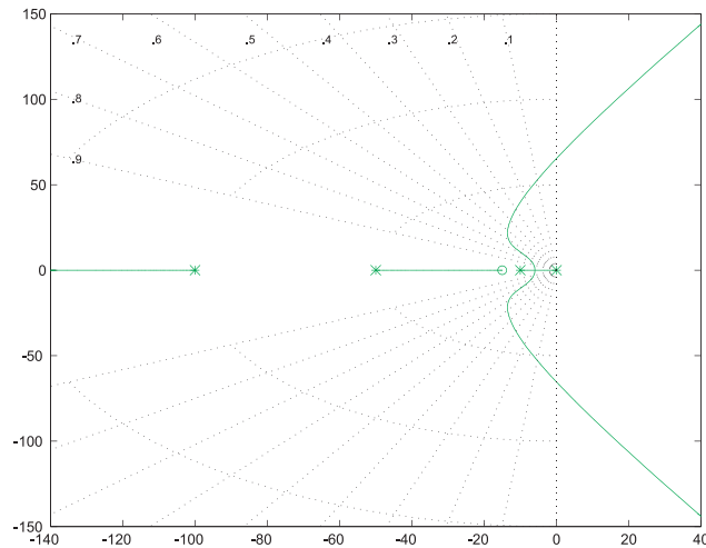
Figura 4.14: Regioni a \delta per G_c(s)G_p(s) .
