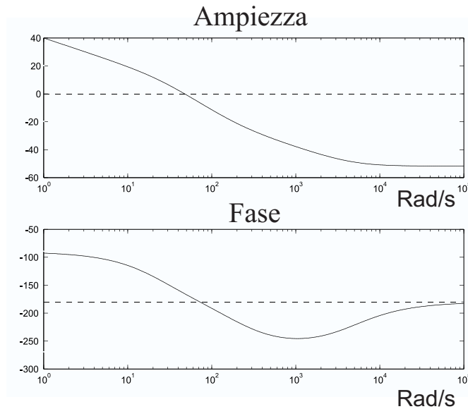
Figura 6.7: Diagrammi di Bode del sistema non compensato.
