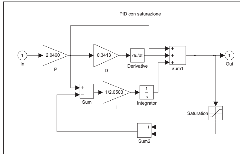
Figura 5.16: Subsystem PID con saturazione in ambiente Simulink .
