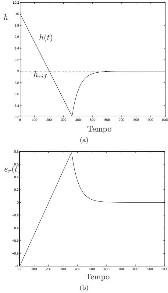
Figura 5.12: Livello del serbatoio e livello di riferimento (a) ed errore a regime (b) con regolatore PI.
