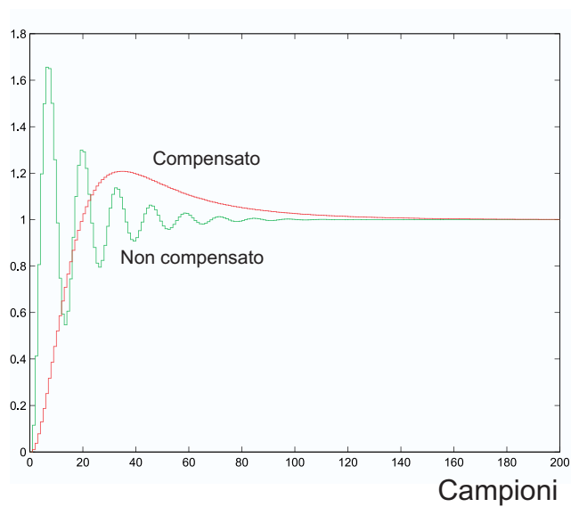
Figura 6.9: Risposta del sistema con e senza compensazione.
