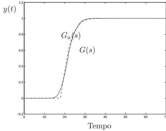
Figura 5.15: Confronto delle risposte al gradino di G(s) e G_a(s) .
