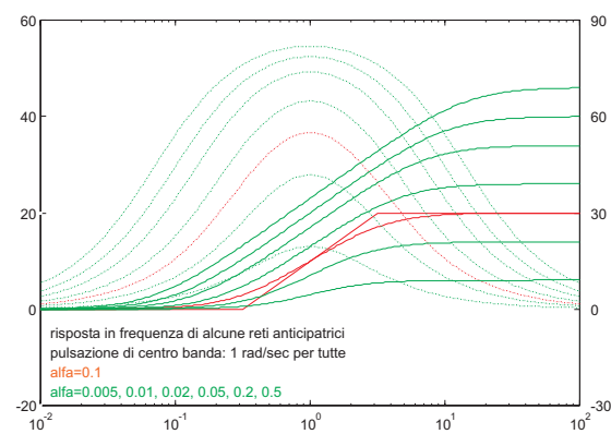
Figura 4.4: Output grafico della funzione leadc .
