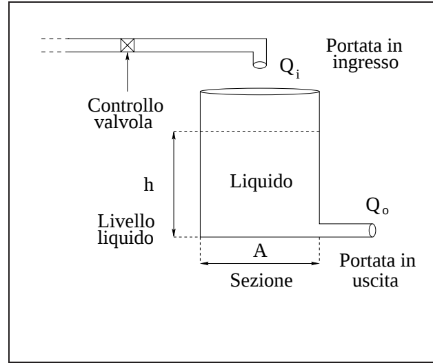
Figura 5.6: Rappresentazione del sistema controllato.
