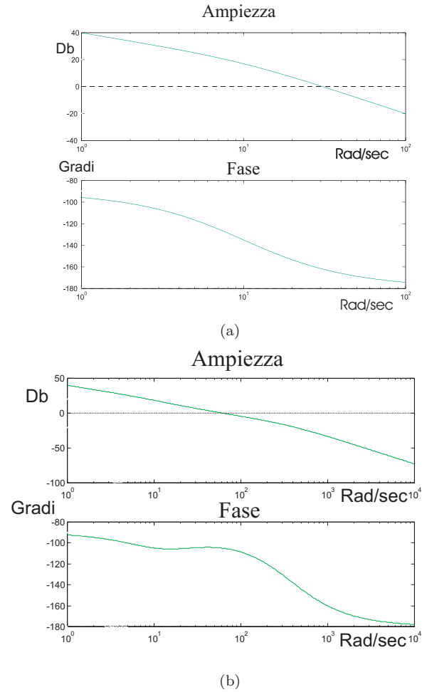
Figura 4.8: Diagrammi di Bode della fase e dell'ampiezza per il sistema non compensato (a) e compensato (b) G_p(s) .
