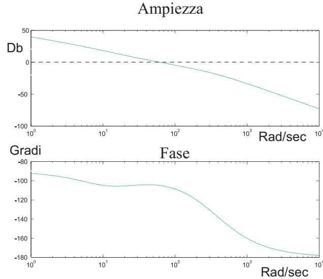
Figura 4.7: Diagramma di Bode della fase e dell'ampiezza per il sistema compensato G(s) = G_c(s) * G_p(s) .
