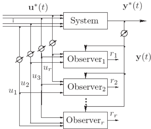
Input sensor FDI
